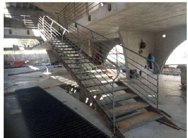
COLOCACION DE ALFARDAS, ESCALONES Y BARANDALES METALICOS DE LAS 2 ESCALERAS INTERIORES DE LA PLANTA BAJA (EJES B/4-5 Y C/2-3)
