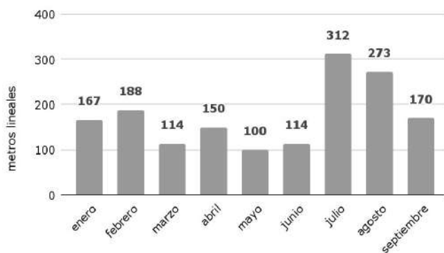
Desazolve de la red de drenaje
