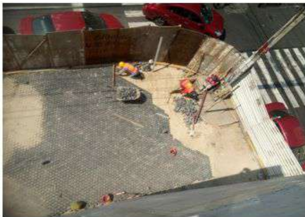
COLOCACIÓN DE PISO DE ADOCRETO CIRCULAR NEGRO DE 10 CM. DE ESPESOR Y 10 CM. DE DIÁMETRO EN PLAZA (EJES 1-7/A-E)
