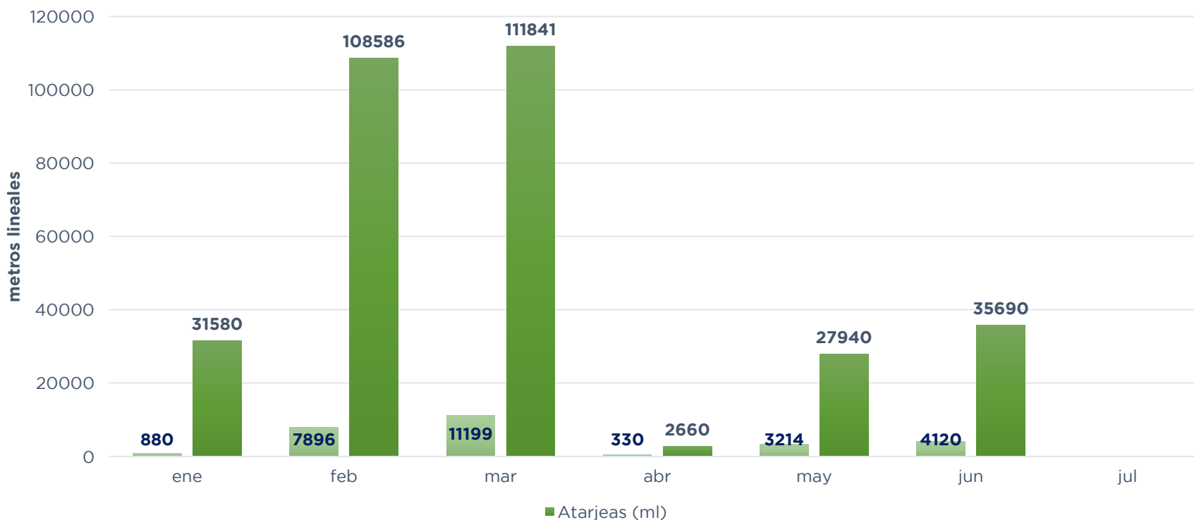
Metraje de red secundaria de drenaje desazolvada
